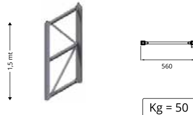
Traliccio piatto - Flat mast - Mât plat
