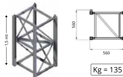
Traliccio quadrato - Square mast - Mât carré
