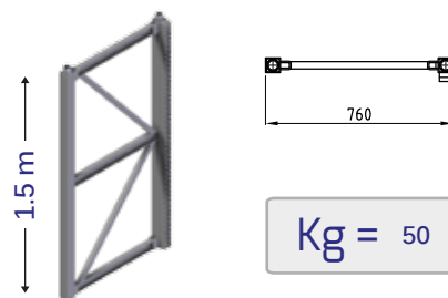
Traliccio piatto Flat mast / Mât plat
